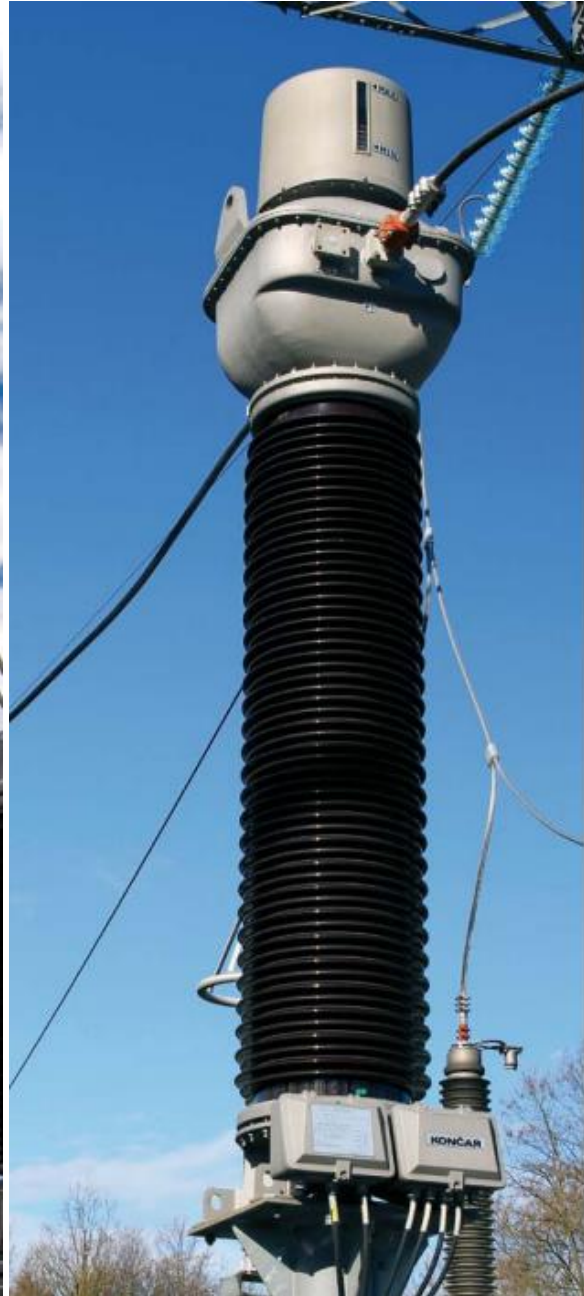
Kombinirani mjerni transformator - tip VAU
